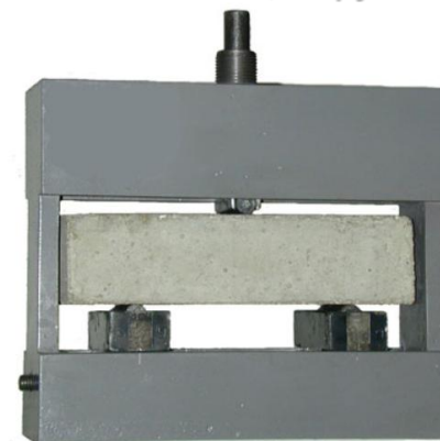
Приспособление к прессу ПИ для испытания на изгиб балочек 40x40x160мм 51 531,0 руб.
